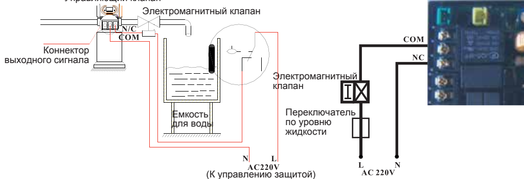
Управляющий клапан
