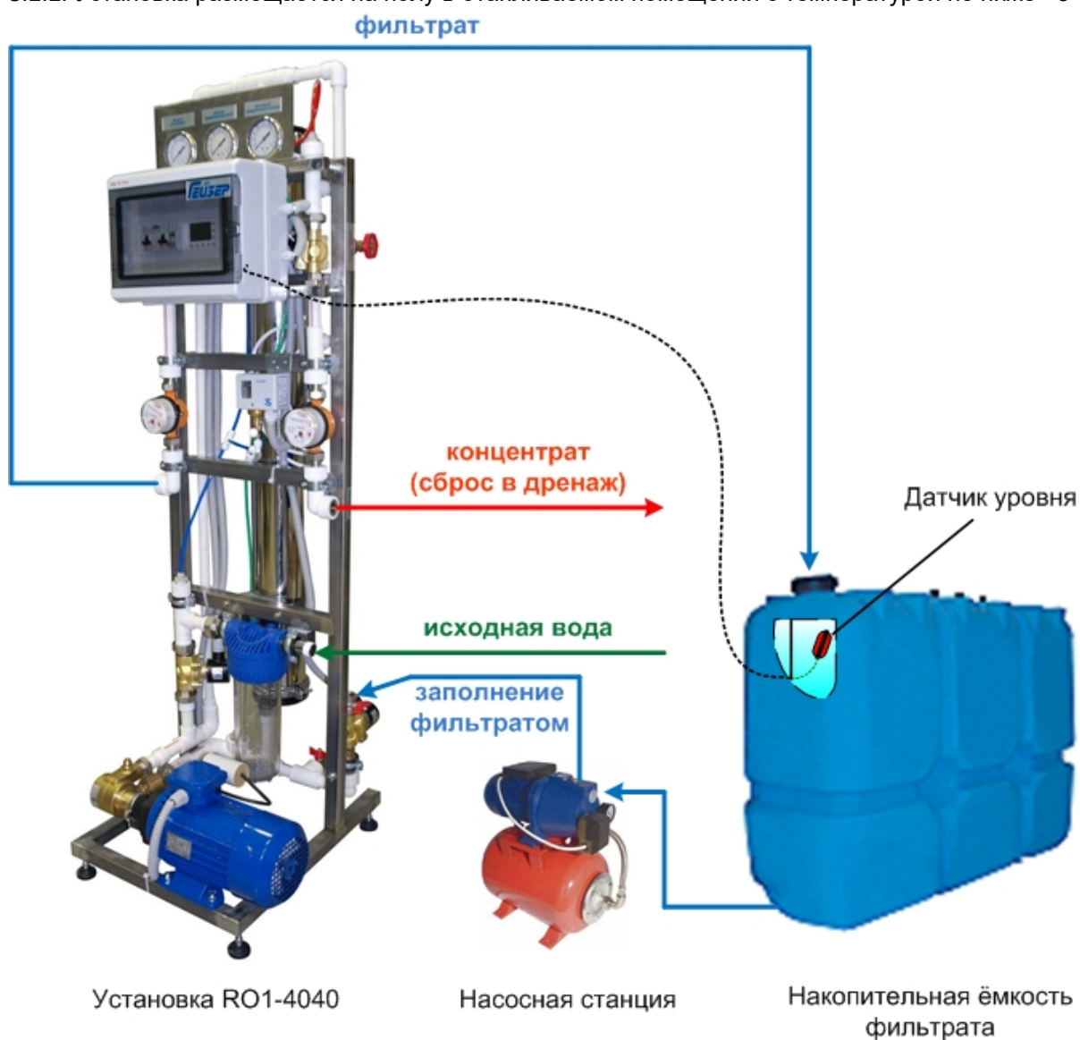
Рис. 4 Подключение трубопроводов к установке.
