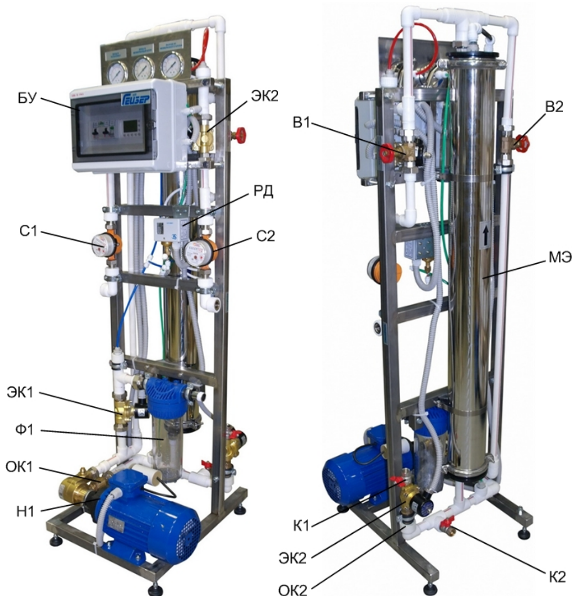
Рис.1 Общий вид установки.
